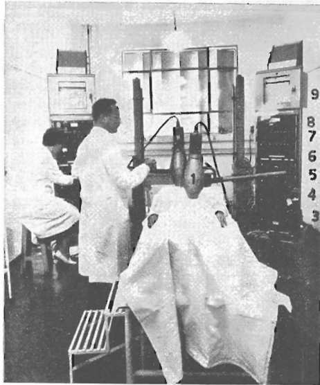
Fig. 4 — Dois sistemas completos de detecção constando de: 1) detector de cintilação com colimador de chumbo; 2) pré-amplificador; 3) fonte de alta tensão; 4) amplificador; 5) analisador de pulsos; 6) «timer» eletrônico; 7) escalímetro; 8) «ratemeter»; 9) registrador gráfico.
