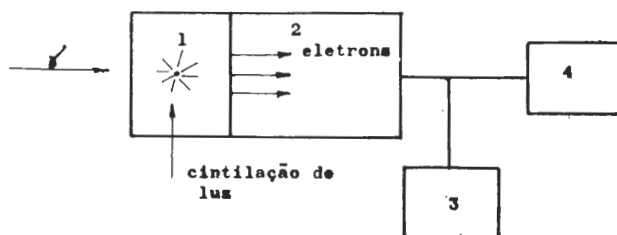
Fig. 3 — Esquema de detector de cintilação: 1) cintilador; 2) válvula fotomultiplicadora; 3) fonte de alta tensão; 4) aparelho de medida.
